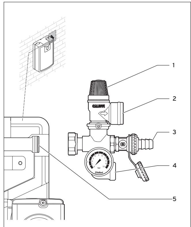
Fig. 5.4 Collegamento del gruppo di sicurezza alla stazione solare
