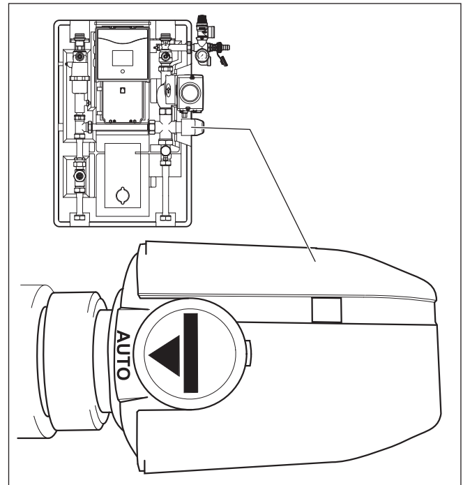
Fig. 5.7 Valvola selettiva
