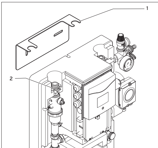
Fig. 5.3 Supporto dell'apparecchio
