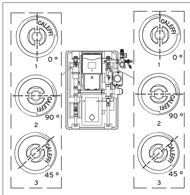
Fig. 10.1 Posizioni della valvola di intercettazione della stazione solare
