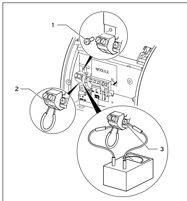
Fig. 10.3 Controllo della resistenza di isolamento
