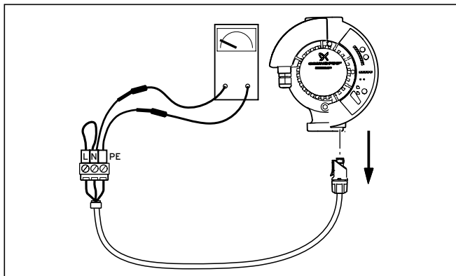
Fig. 10.2 Prova del cavo di collegamento
