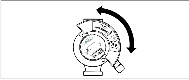
Fig. 4.4 Rotazione di statore e testa della pompa
