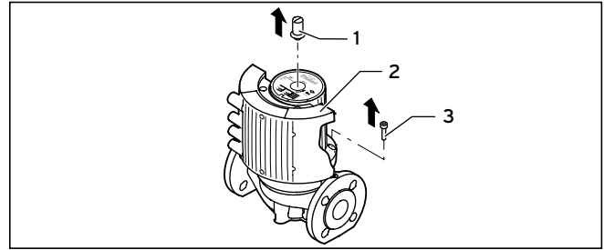
Fig. 4.5 Disimpegno dell'alloggiamento dello statore
