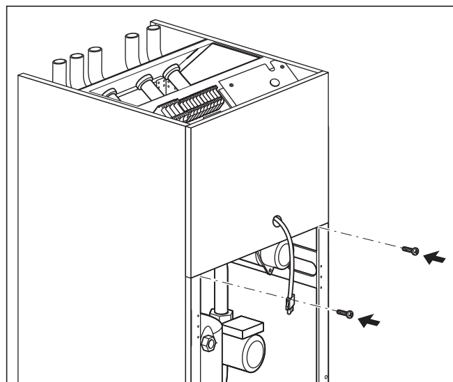
Fig. 6.21 Montaggio del rivestimento anteriore superiore
