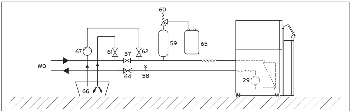
Fig. 5.1 Circuito della miscela incongelabile
