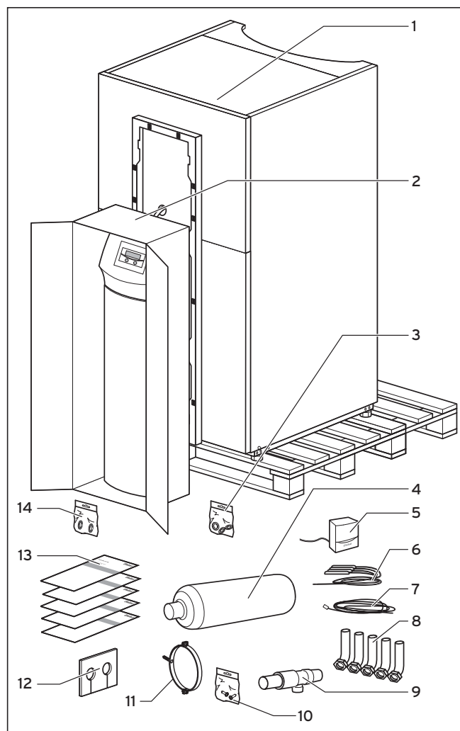
Fig. 4.4 Controllo della fornitura
