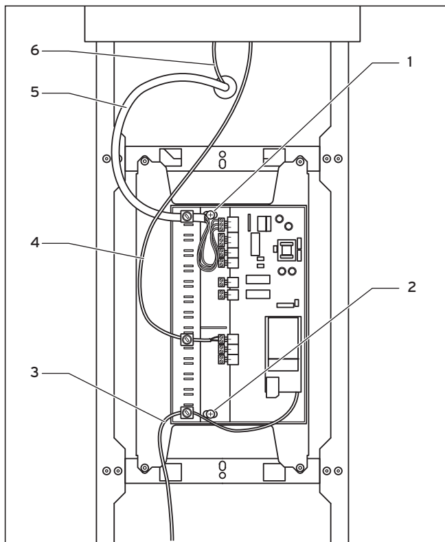
Fig. 6.18 Installazione di vnetDIALOG
