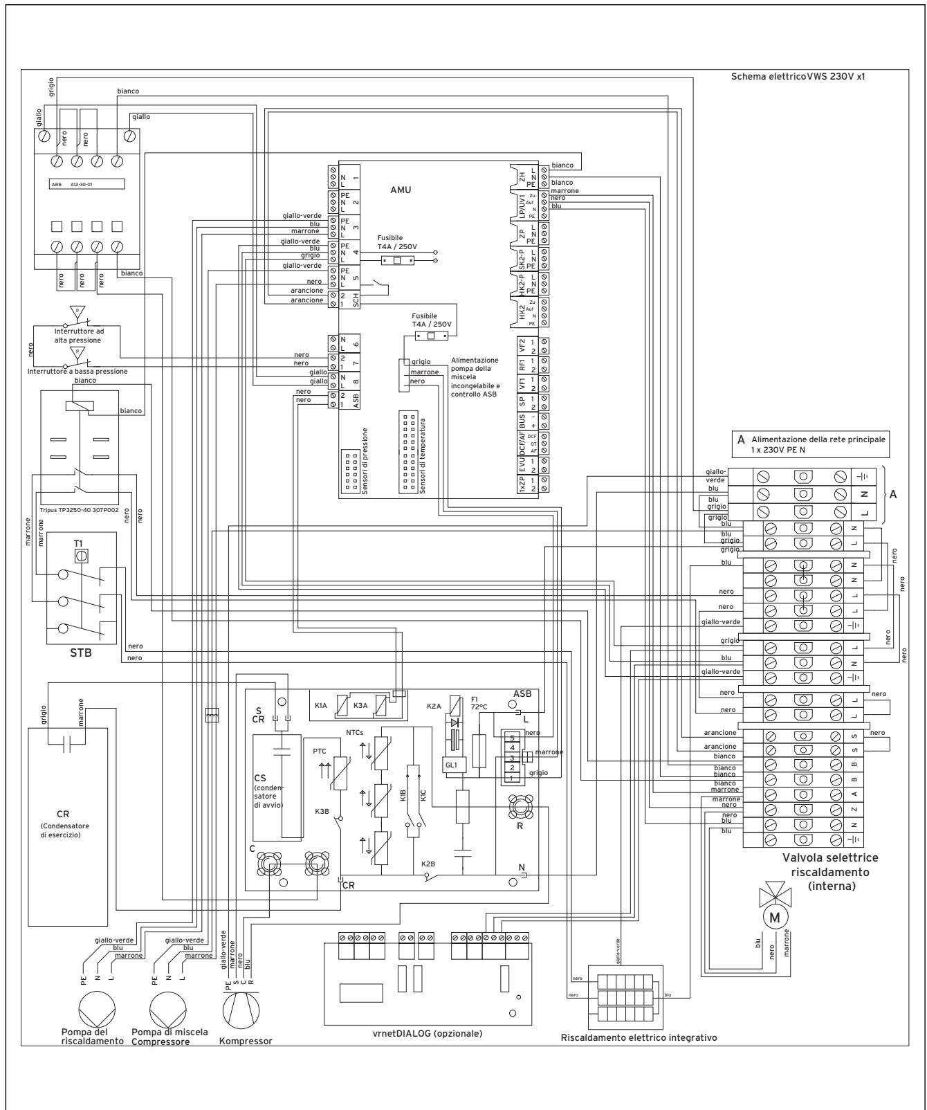
Fig. 2 Appendice, schema elettrico
