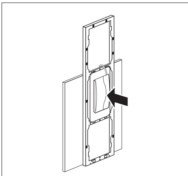
Fig. 6.17 Montaggio di vnetDIALOG
