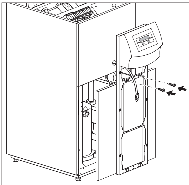
Fig. 6.23 Montaggio del rivestimento anteriore inferiore
