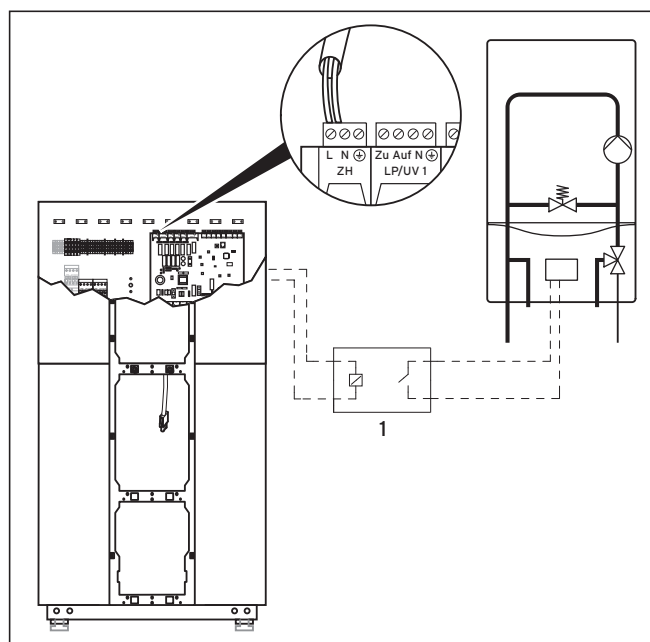
Fig. 6.20 Collegamento del riscaldatore senza interfaccia eBUS
