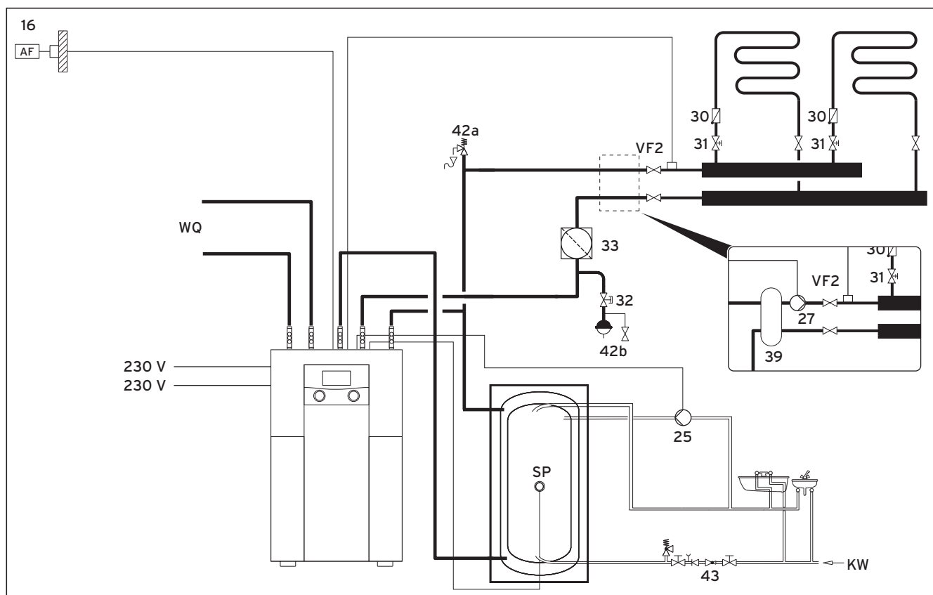
Fig. 6.11 Schema idraulico 3
