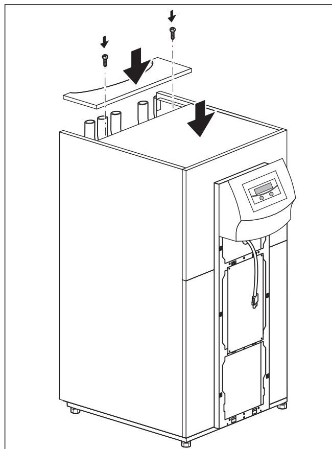
Fig. 6.24 Montaggio della copertura superiore
