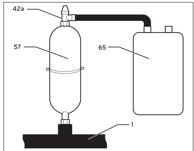
Fig. 4.14 Montaggio del serbatoio di compensazione miscela incongeloabile
