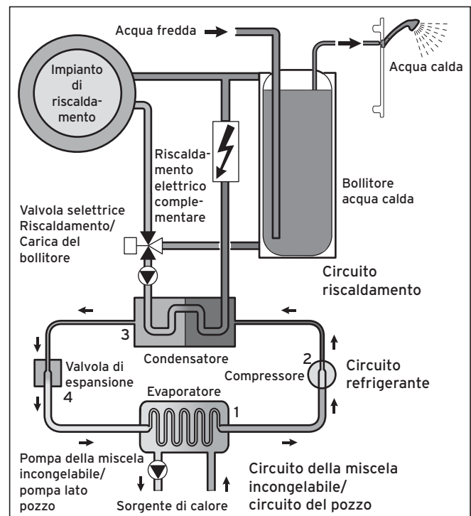
Fig. 3.3 Modalità di funzionamento della pompa di calore
