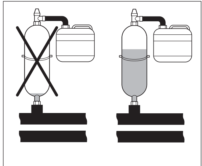
Fig. 6.1 Livello del serbatoio di compensazione della miscela incongelabile
