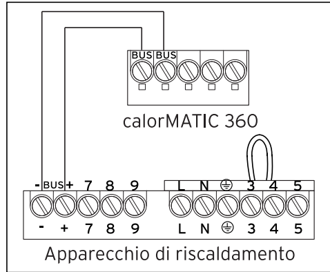
Fig. 10.1 Allacciamento elettrico
