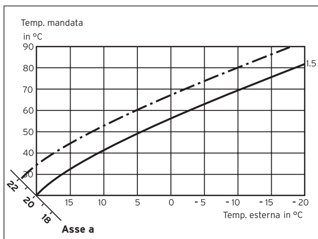
Fig. G.2 Spostamento in parallelo della curva di riscaldamento
