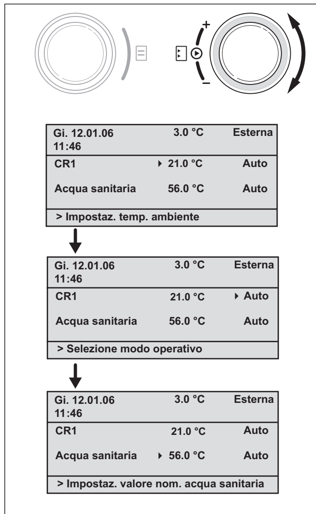
Fig. 4.5 Passaggio da un parametro modificabile a un altro
