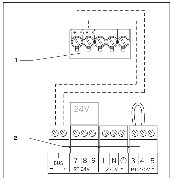
Fig. 5.1 Collegamento elettrico di calorMATIC 430
