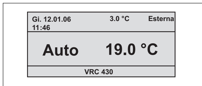
Fig. 4.8 Schermata di base semplificata (esempio)
