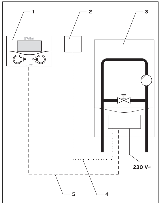
Fig. 2.1 Schema del sistema
