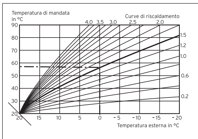
Fig. G.1 Diagramma con curve di riscaldamento per una temperatura ambiente nominale di 20 °C
