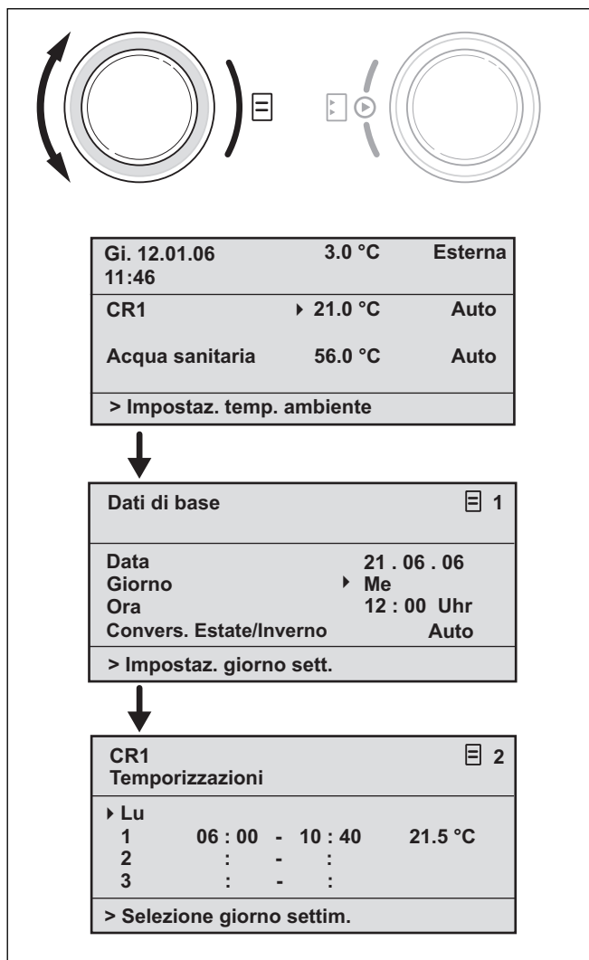
Fig. 4.4 Visualizzazione di altre schermate
