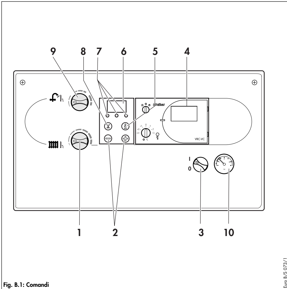
Fig. B.1: Comandi
