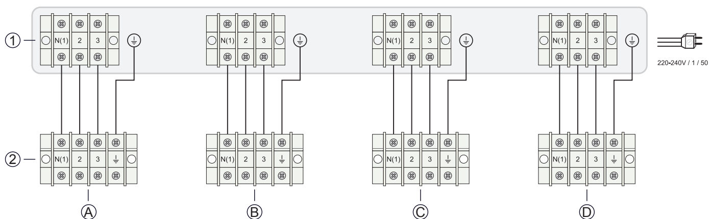
Fig. 11.4 Schema elettrico per il collegamento tra le unità esterna e interna.
