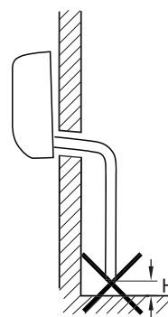
Fig. 9.4 Distanza minima dal pavimento.
