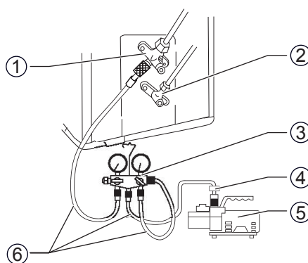
Fig. 12.2 Spurgo dell'impianto.
