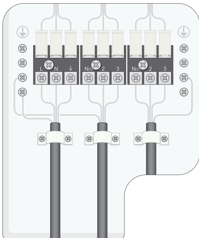
Fig. 11.2 Collegamento elettrico dell'unità esterna 3-060 W2NO.
