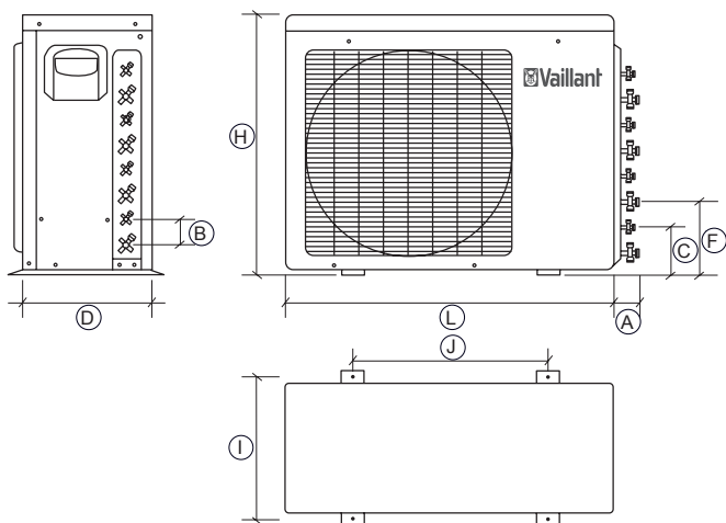
Fig. 5.3 Dimensioni dell'unità esterna.
