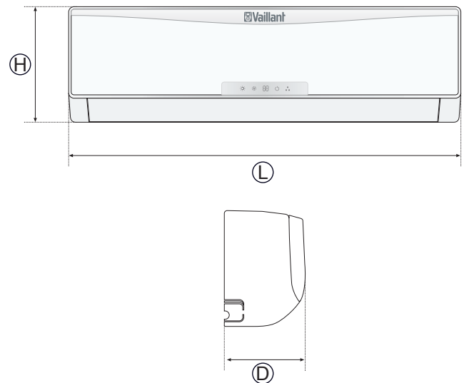
Fig. 5.2 Dimensioni dell'unità interna.
