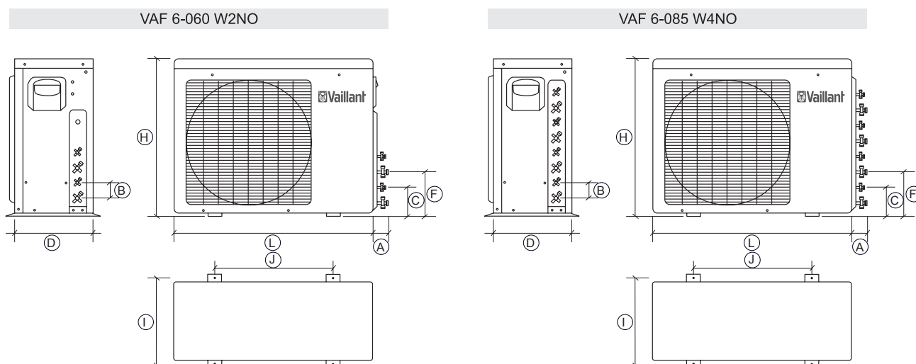
Fig. 5.3 Dimensioni dell'unità esterna.
