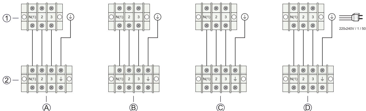
Fig. 11.3 Schema elettrico per il collegamento tra le unità esterna e interna
