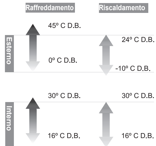
Fig. 2.1 Intervalli di funzionamento dell'unità.
