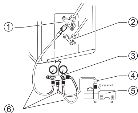
Fig. 12.2 Spurgo dell'impianto.
