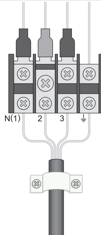
Fig. 11.1 Collegamento elettrico dell'unità interna.
