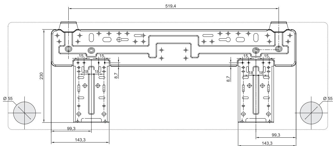
Fig. 9.6 Piastra di sostegno per l'unità VAI 6-025 WMNI.
