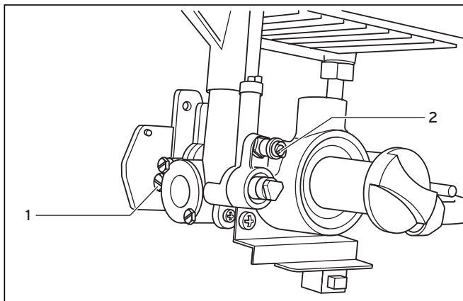
Fig. 6.1 Bocchettoni per la misurazione della pressione di allacciamento del gas
