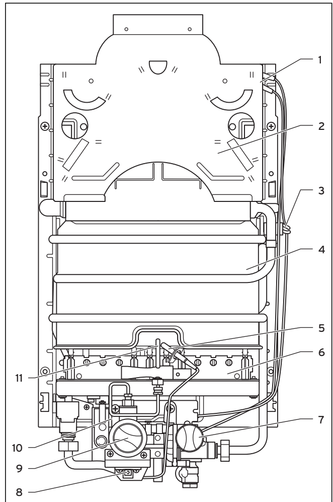
Fig. 2.1 Gruppi costruttivi tipo (Y) XZ
