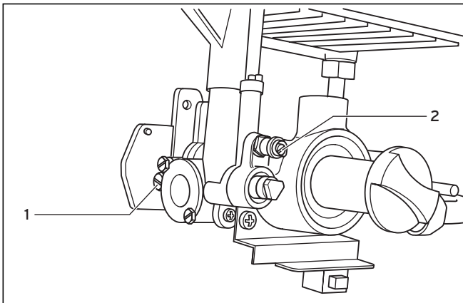
Fig. 6.4 Bocchettone per la misurazione della pressione del bruciatore
