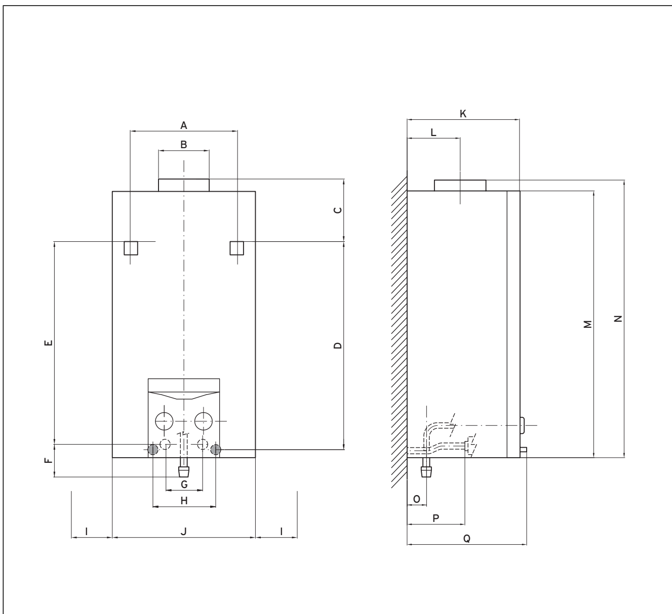
Fig. 4.3 Dimensioni mini 11-0/0 XZ metano
