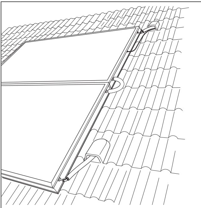
Figura 2.4 Campo a 2 collettori auroTHERM classic VFK 135 D con montaggio su tetto
