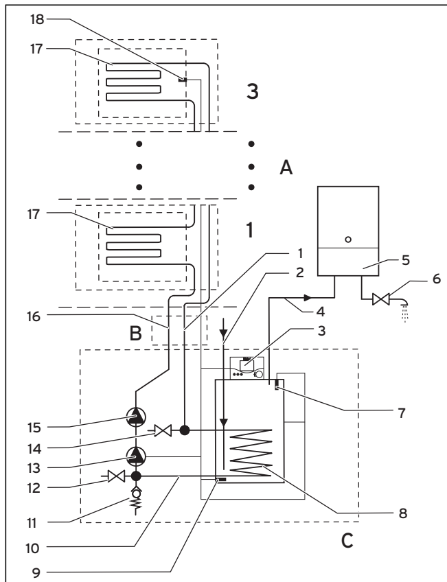
Figura 2.3 Componenti principali del sistema auroSTEP plus con bollitore VIH SN 150/3 MiP (disegno di massima, senza accessori per il collegamento)
