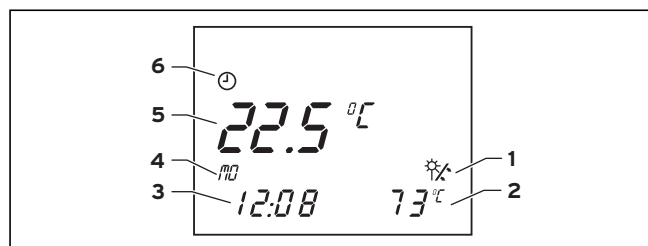
Fig. 4.4 Display livello di comando principale
