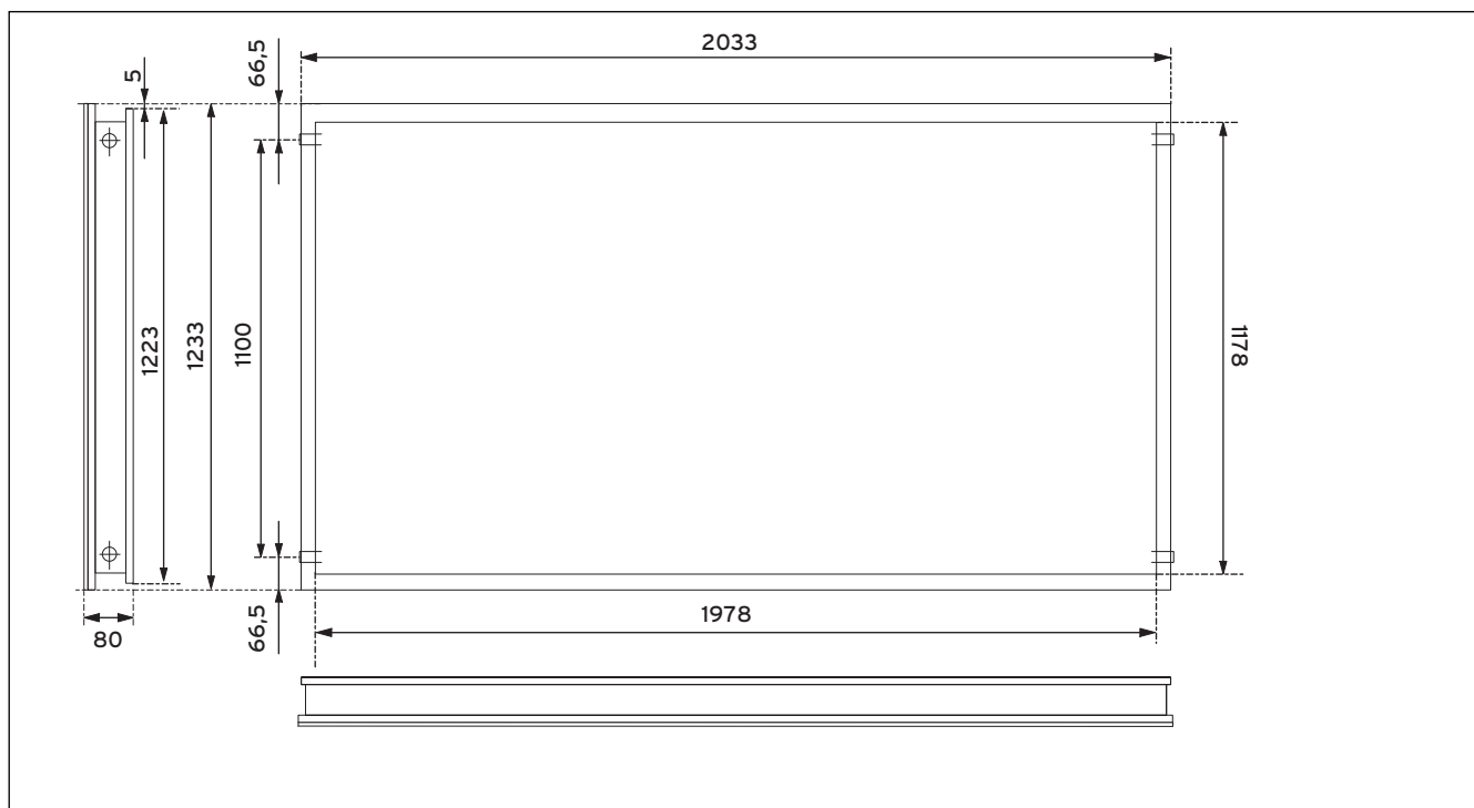
Fig. 12.2 Disegno quotato VFK 145/2 H, VFK 155 H
