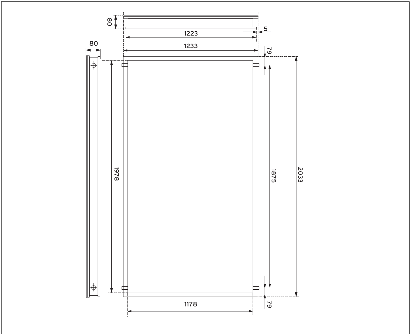
Fig. 12.1 Disegno quotato VFK 125/3, VFK 145/2 V, VFK 155 V
